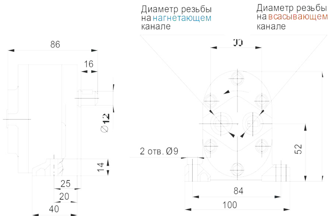
Насос Г11-1
