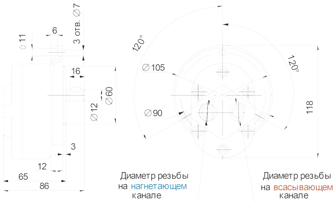
Насос АГ11-11Х
